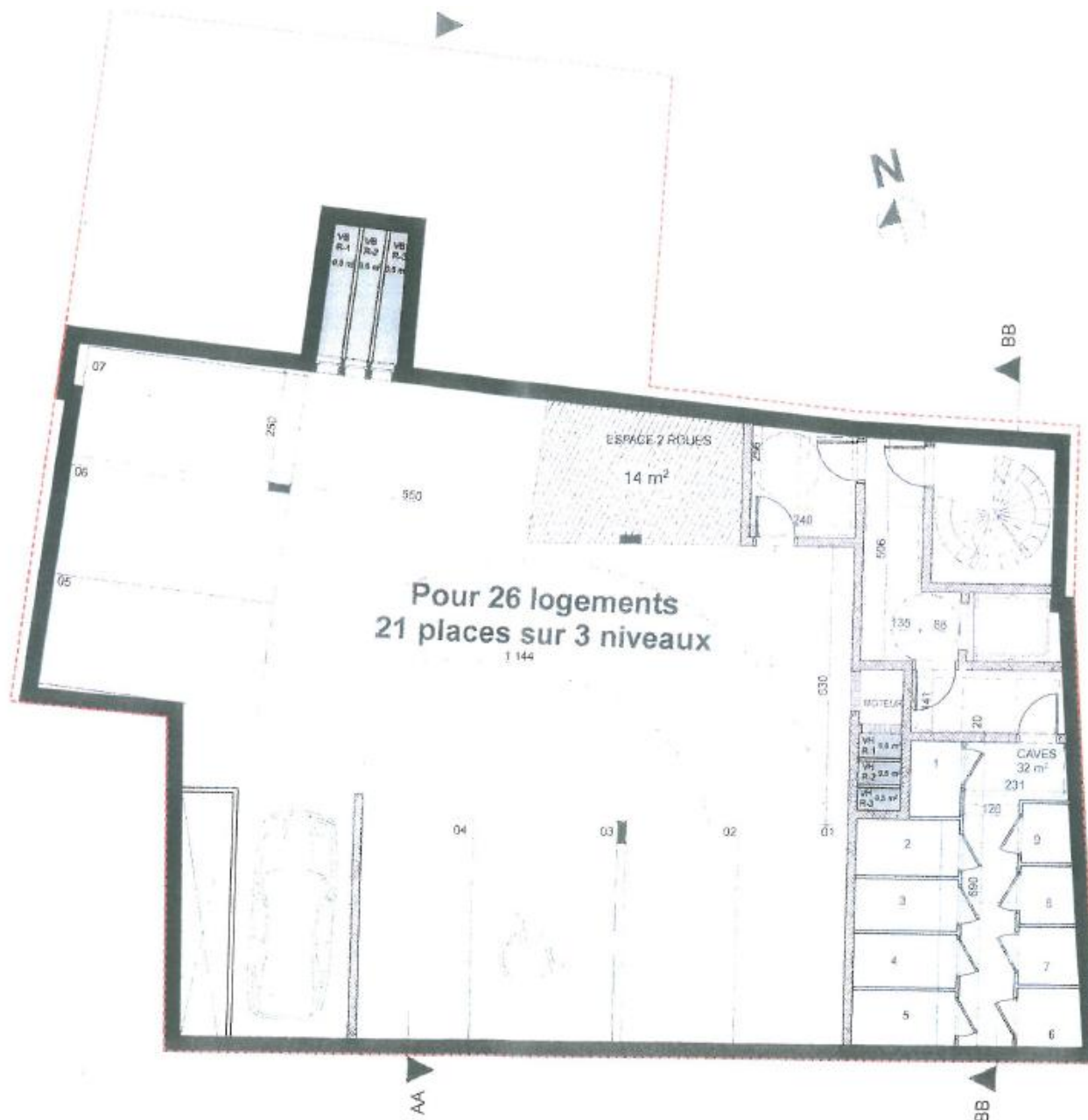
4-6 RUE ADELAIDE LAHAYE - 93170 BAGNOLET PLAN 1er SOUS-SOL
